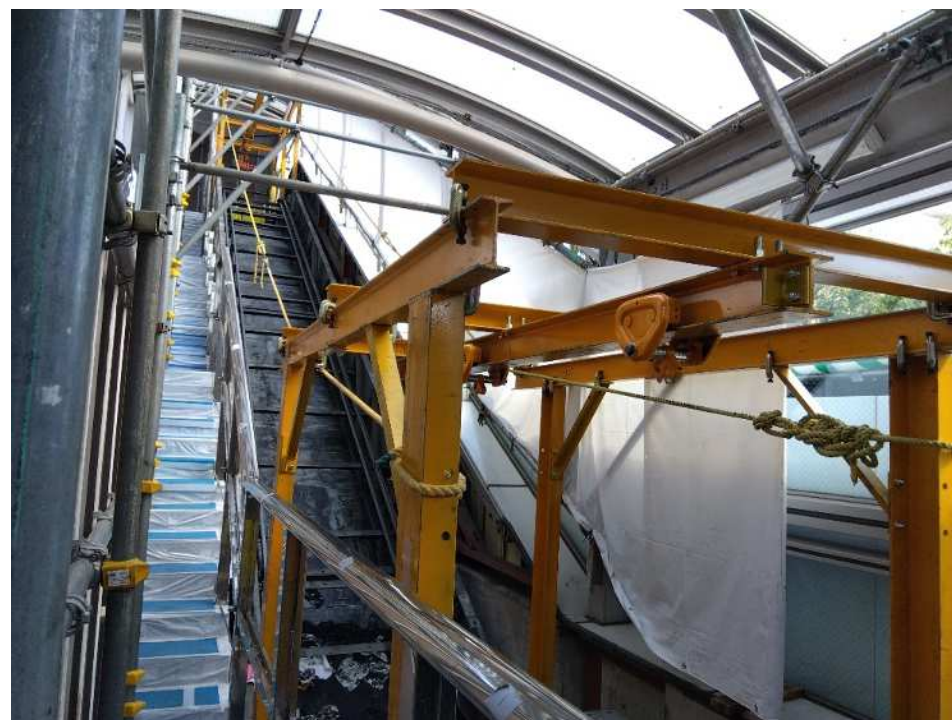
既存エスカレーター 解体状況
