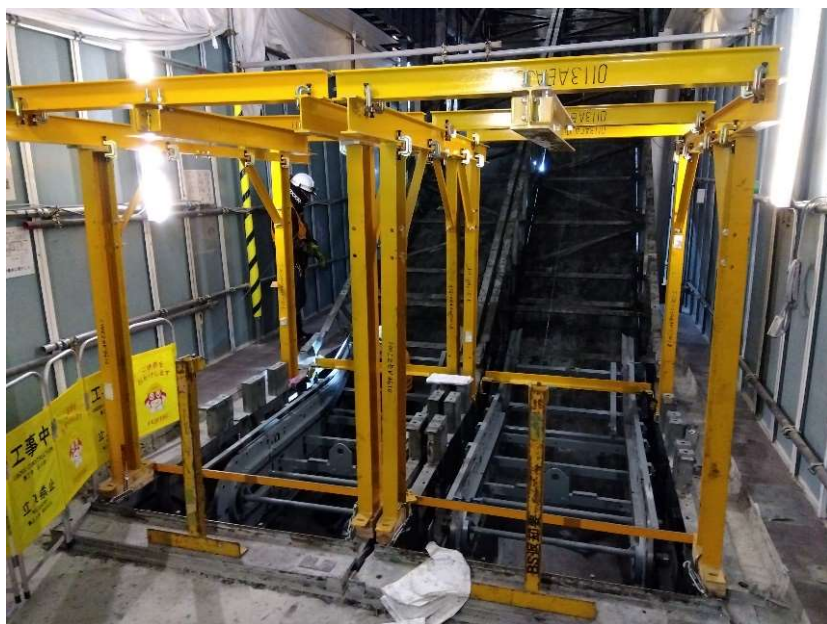
部品の撤去・設置用の吊り台
